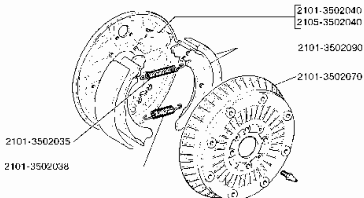
35 02. Тормоза задние
