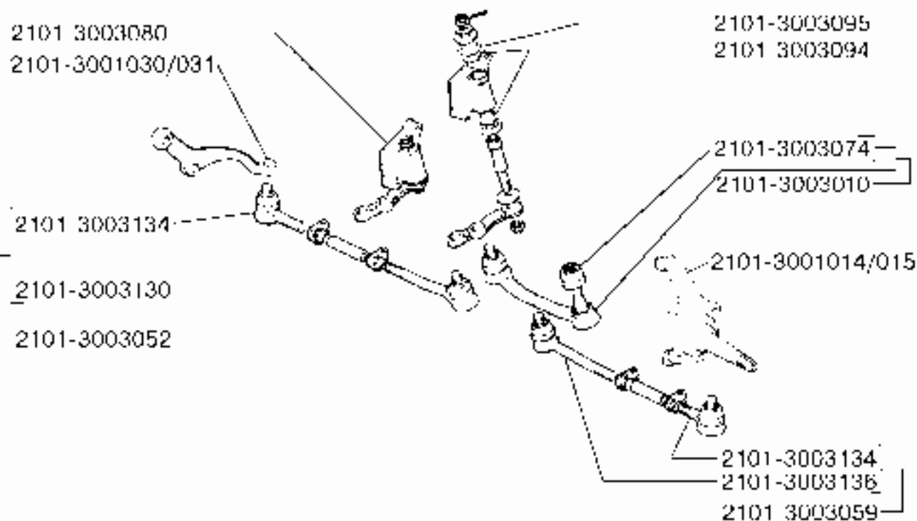
30 00. Кулаки поворотные и тяги рулевые
