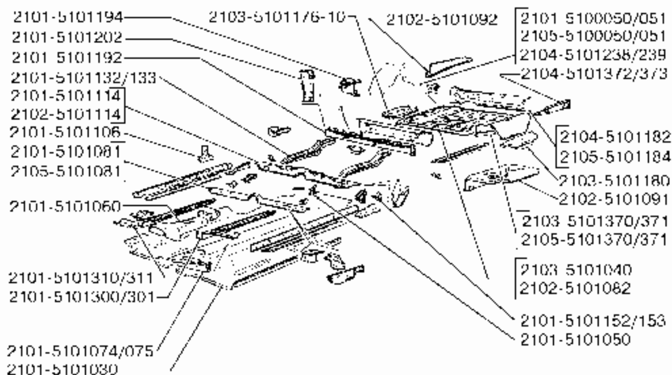
51 01. Детали пола кузова
