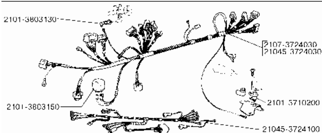
37 24. Жгуты проводов
