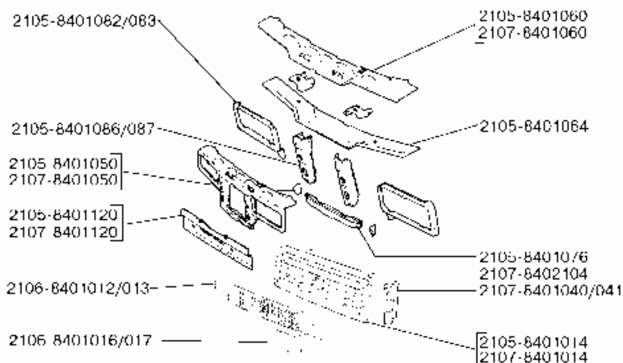
84 01. Облицовка и рамка радиатора
