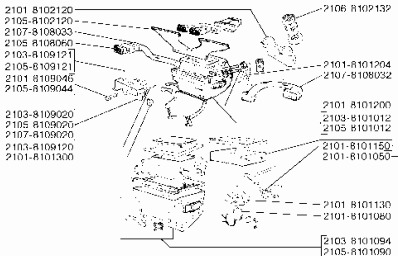
81 01. Отопитель
