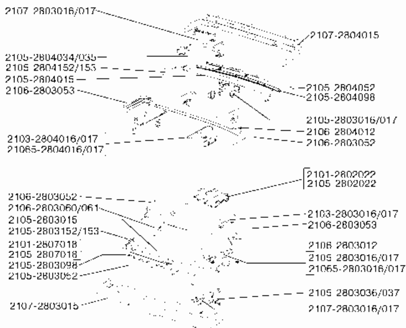
28 00. Защитные элементы кузова
