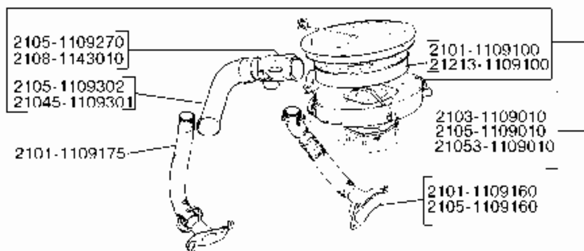
11 09. Фильтр воздушный
