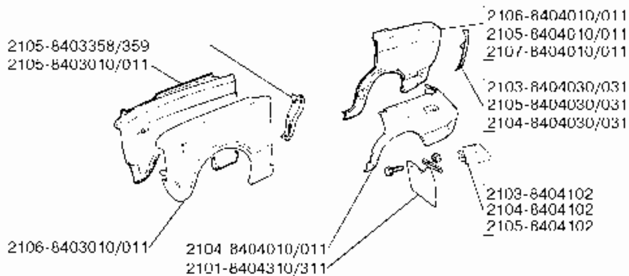
84 03, 84 04. Крылья передние и задние
