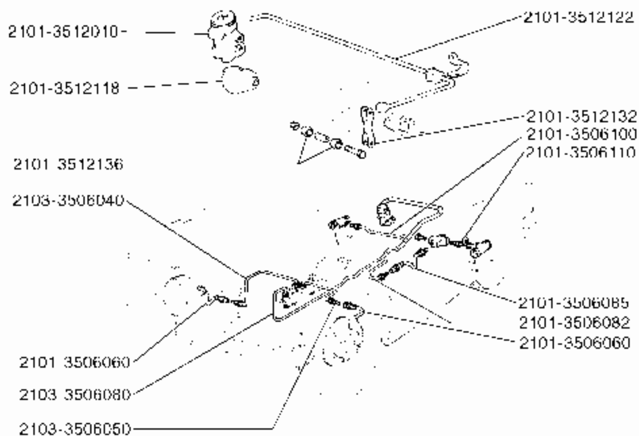
35 06. Трубопроводы тормозной системы
