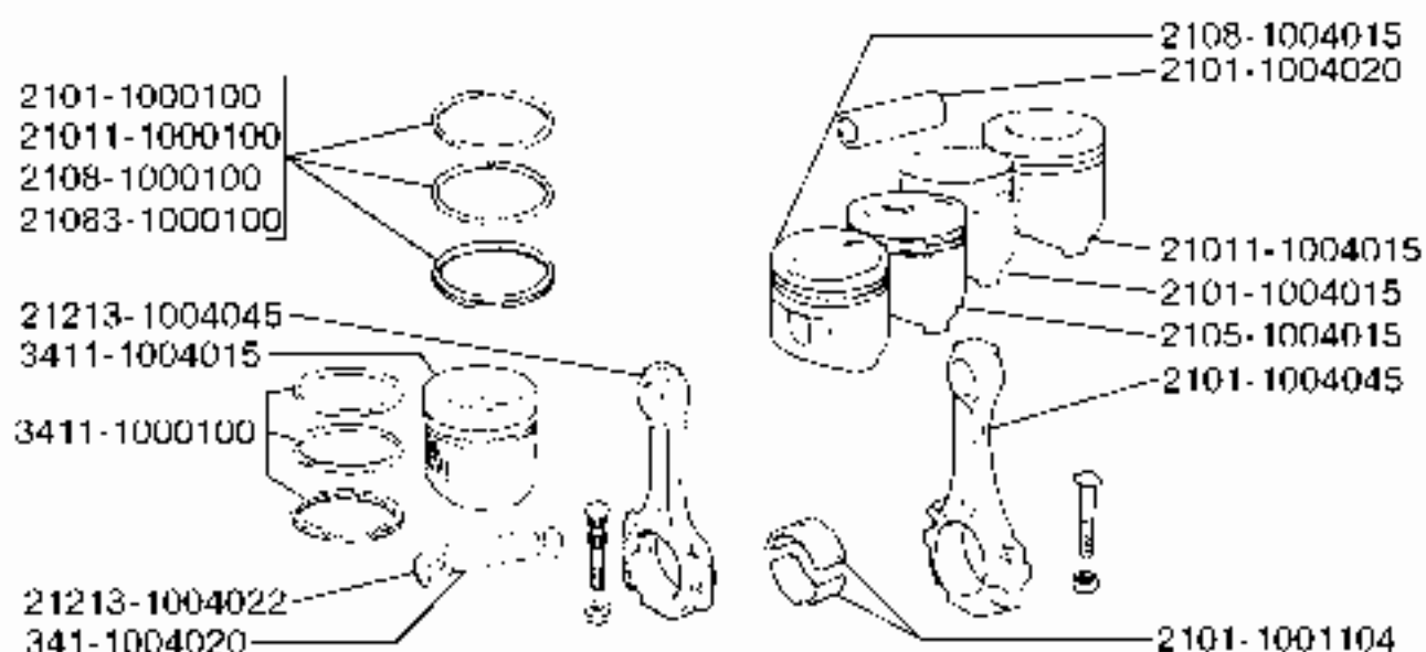
10 04. Поршни и шатуны
