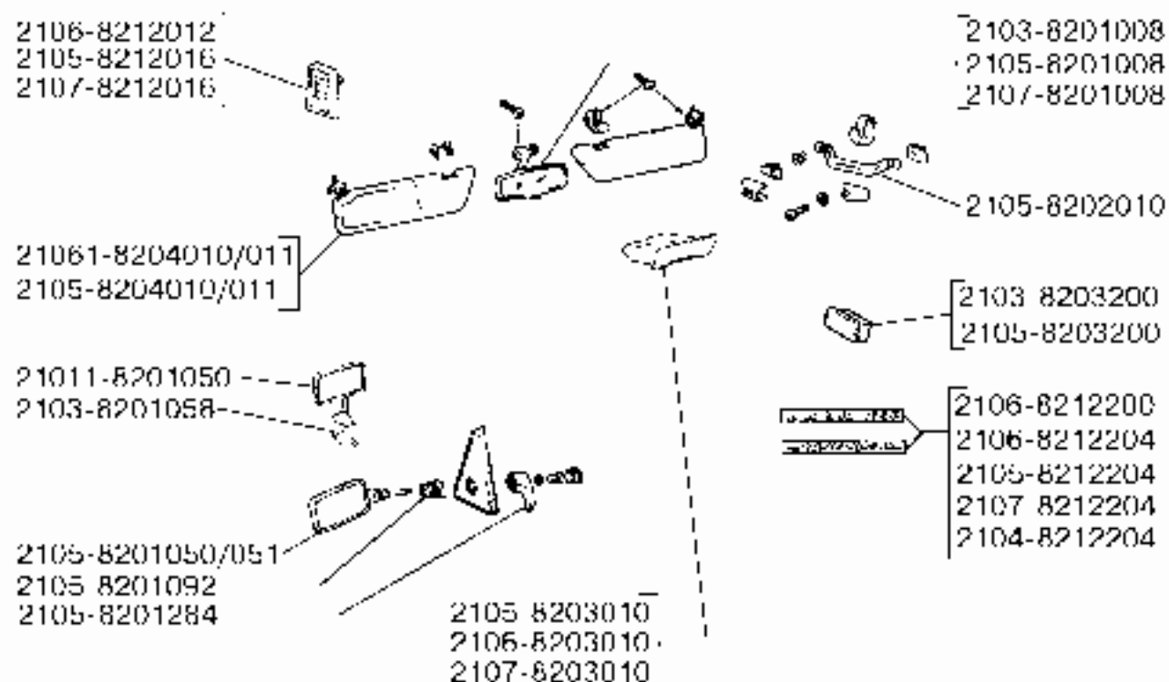
82. Принадлежности кузова
