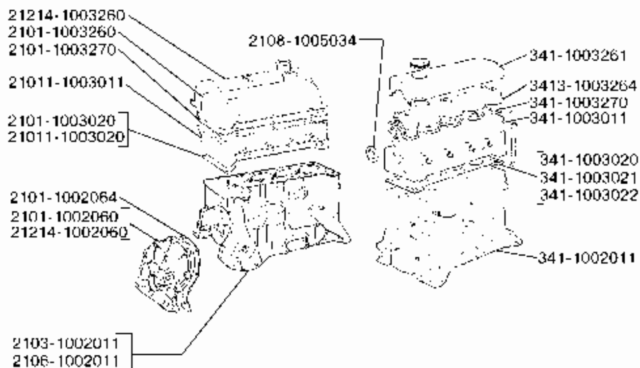
10 02. Блок цилиндров
