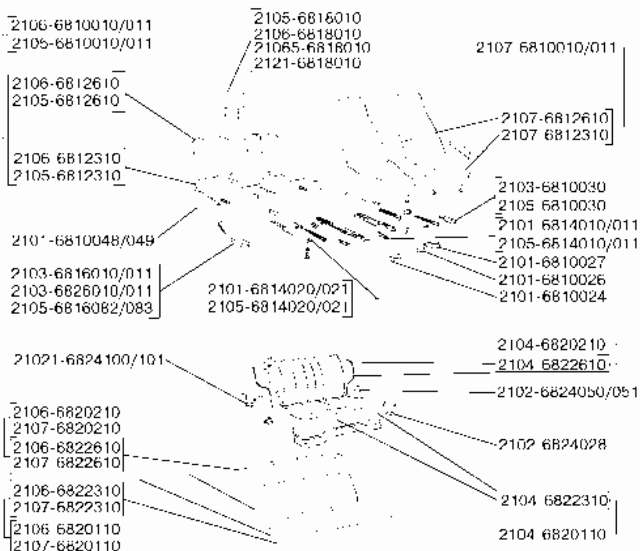
68. Сиденья передние и задние
