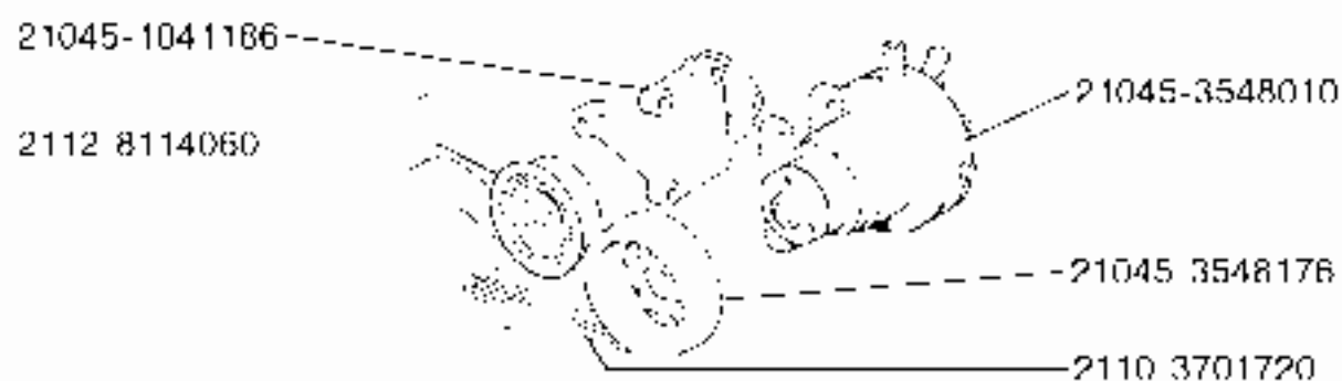
35 48. Насос вакуумный и его привод
