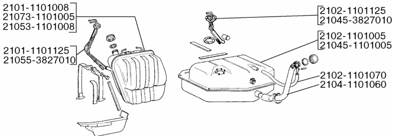
11 01. Бак топливный
