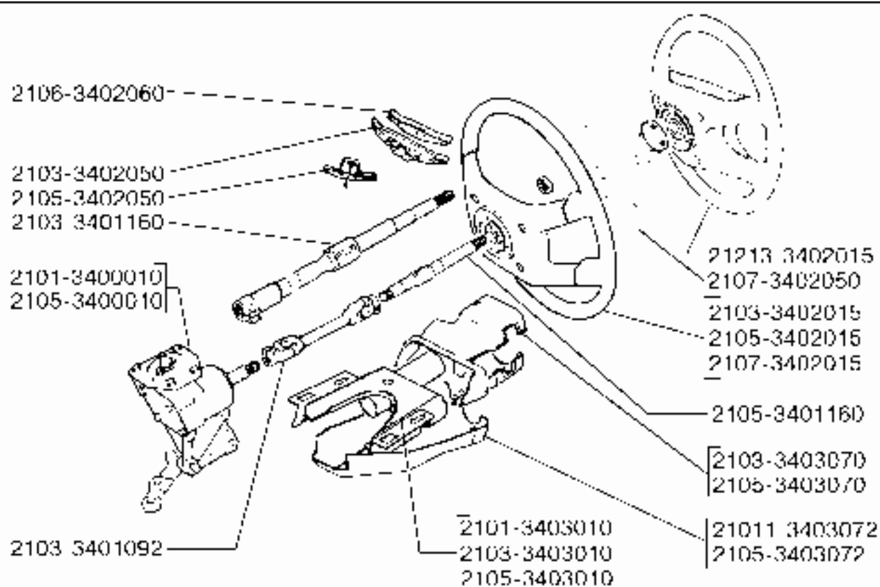
34 00. Управление рулевое
