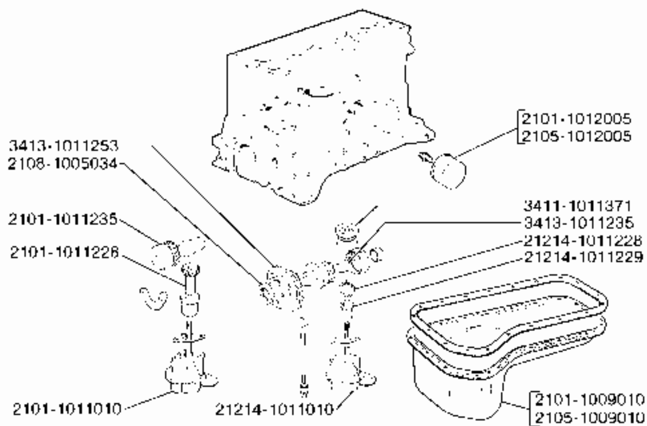
10 09. Картер масляный
