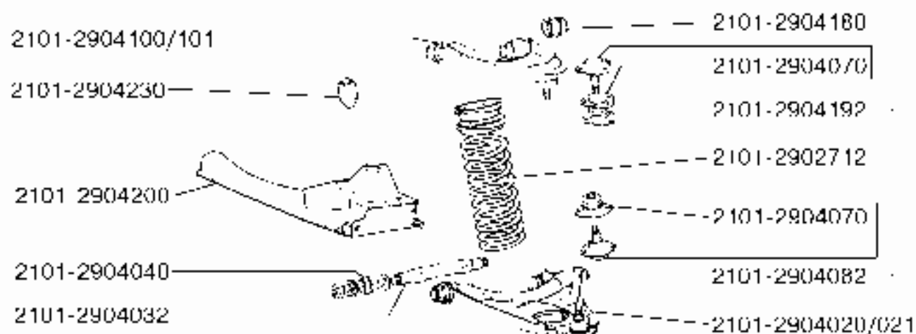
29 01. Подвеска передняя
