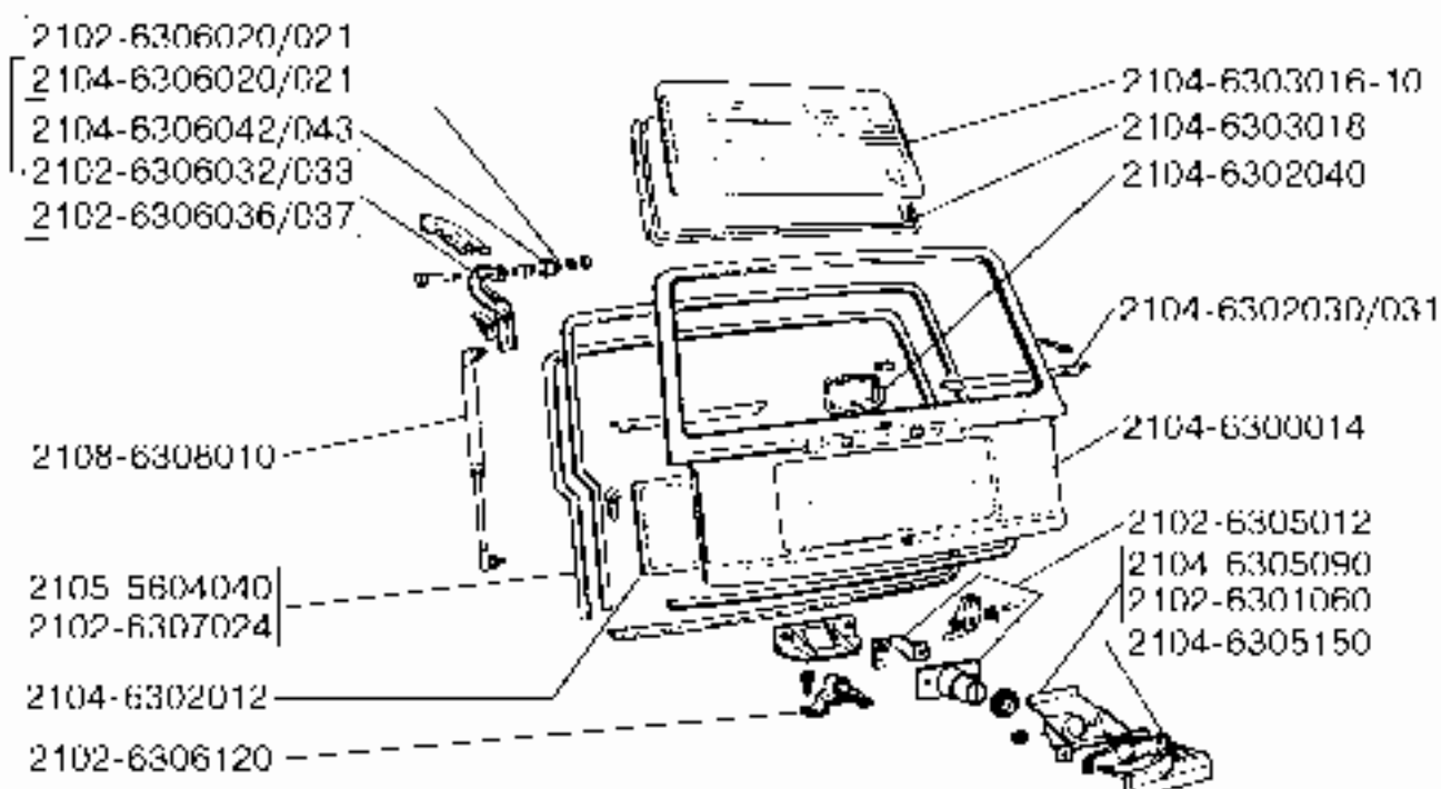
63 00. Дверь задка
