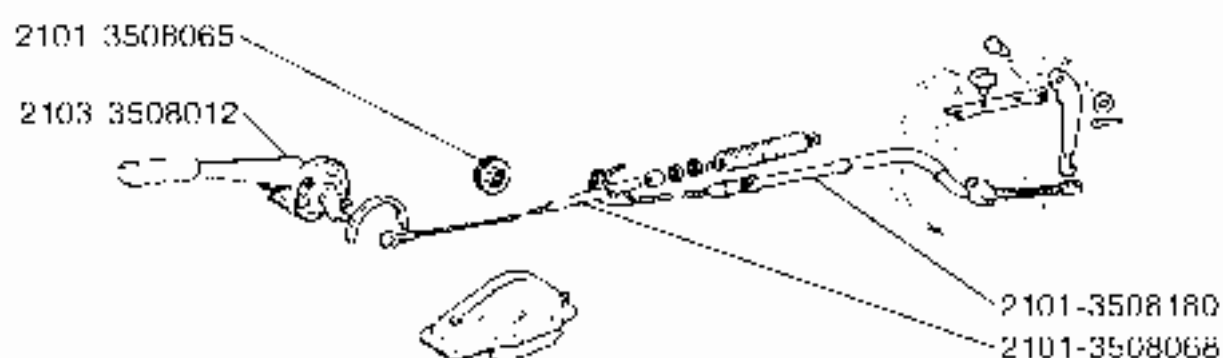
35 08. Управление стояночным тормозом
