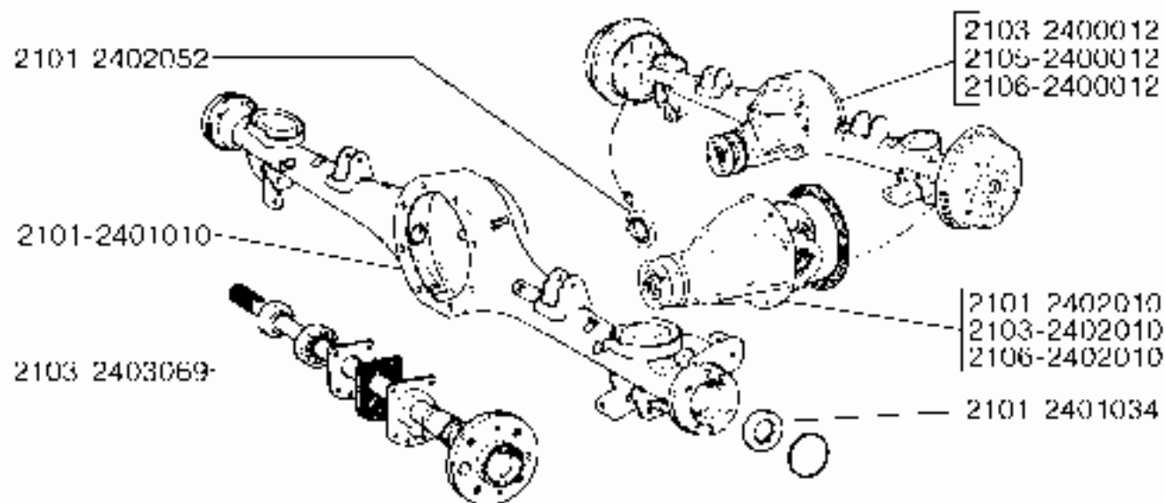
24 00. Мост задний
