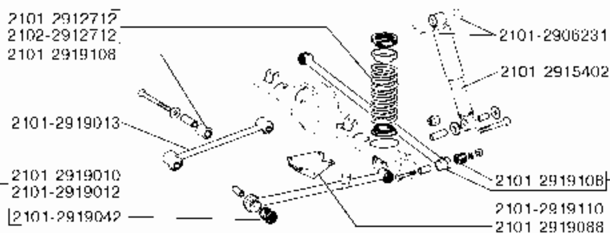
29 15. Амортизаторы задней подвески
