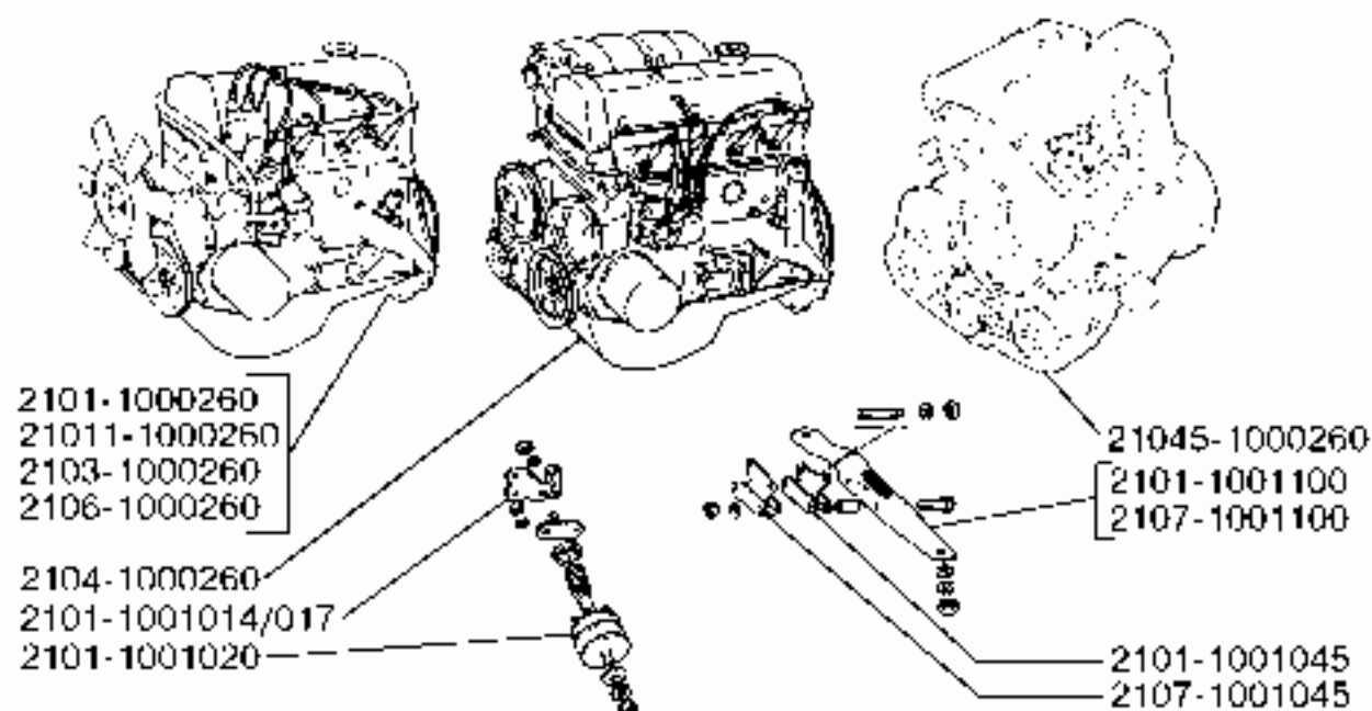
10 00. Двигатель в сборе
